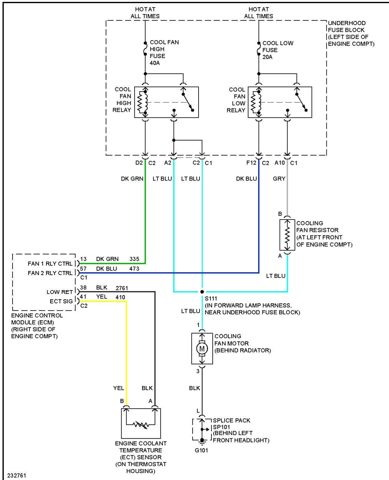
Fig. 12: 2.2L VIN D, Cooling Fan Circuit
