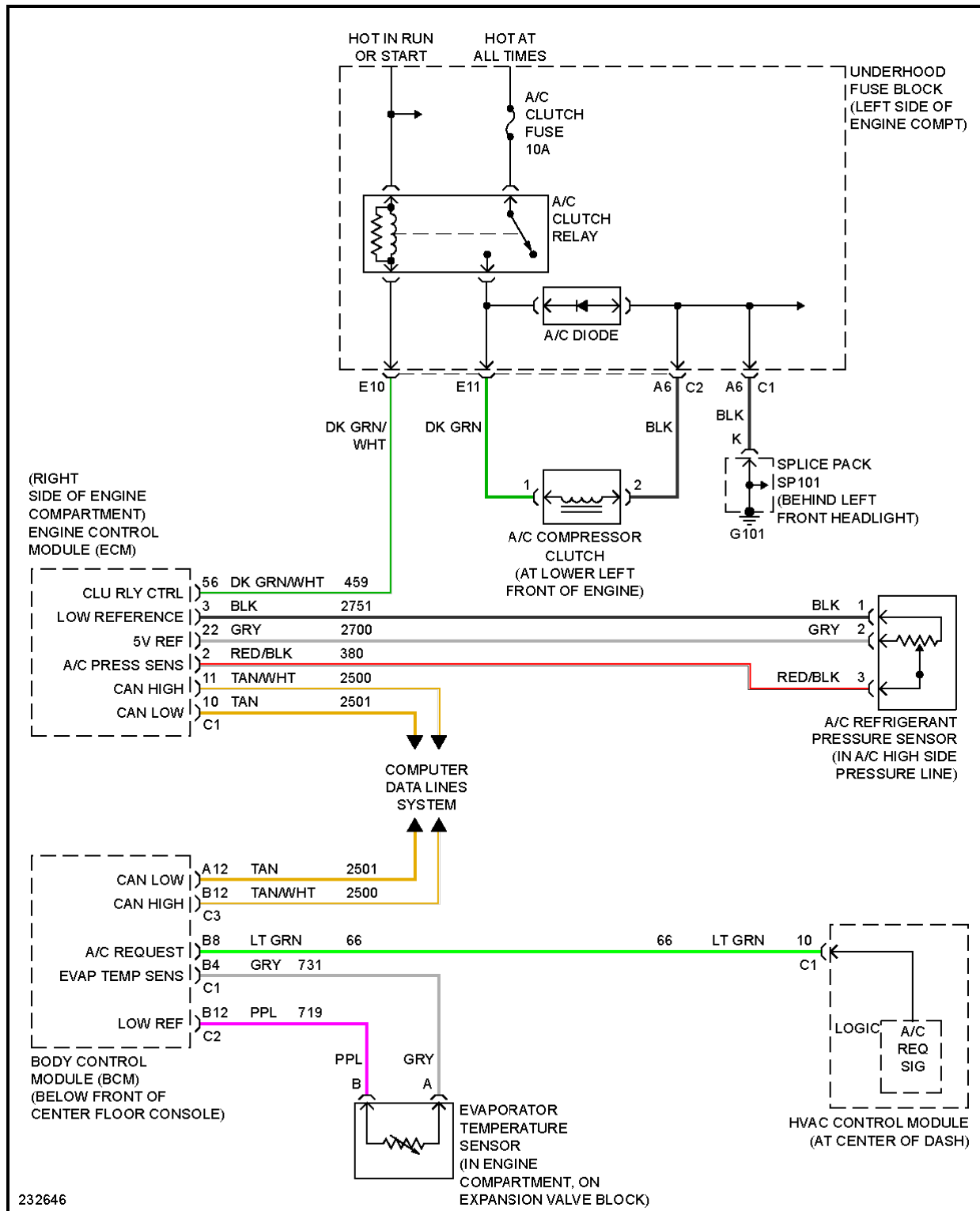
Fig. 1: 2.2L VIN D, Compressor Circuit
